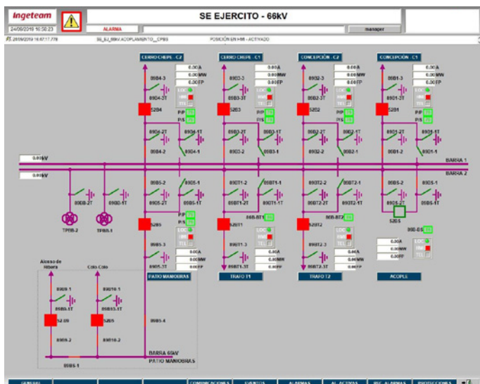
ALARME ALARME MENSAGEM 22/04/2025 20:22:149.444 - 000V 1L 100 23.000 FALSA COMBUSTIVO ALARME ESTADOS SELECTOR LOCAL DESJUNTOR SELECTOR LOCAL SEC. BARRAS SELECTOR LOCAL SEC. LINHA SELECTOR LOCAL SEC. INTERBARRAS SENA 2
